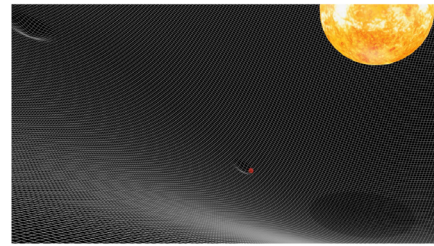
太陽と水星の重力井戸（メッシュで表示）を通過する探査機（赤丸）のイメージ図
